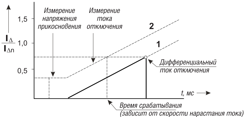
Риc. 30 Зависимости нарастания значения тока от времени птн определении минимального отключающего дифференциального тока УЗО
