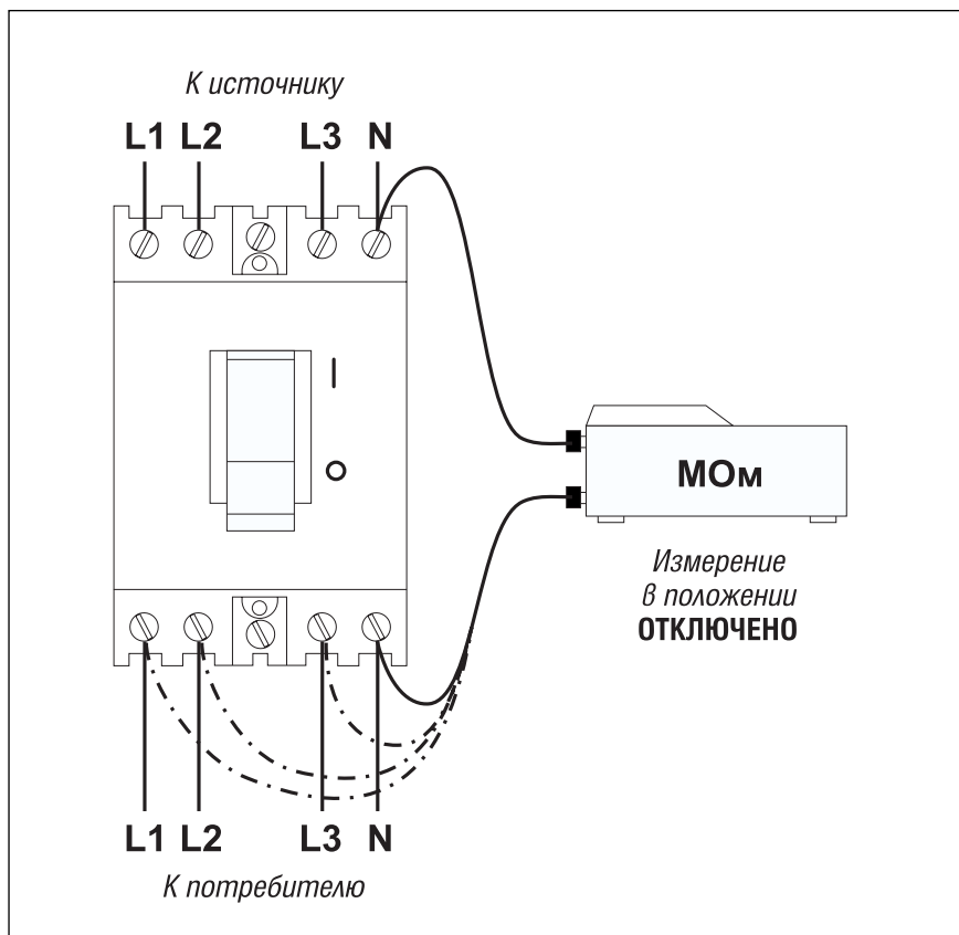
Риц. 28 Измерение сопротивления изоляции в цепи с УЗО
